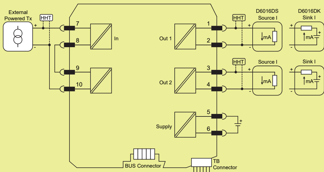
D6016D* Duplicator
