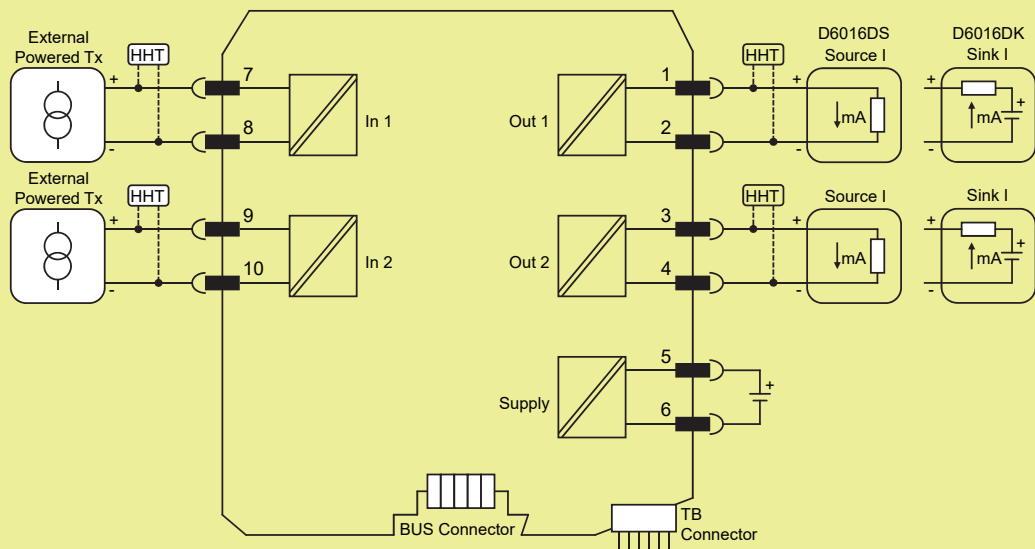
D6016D*
