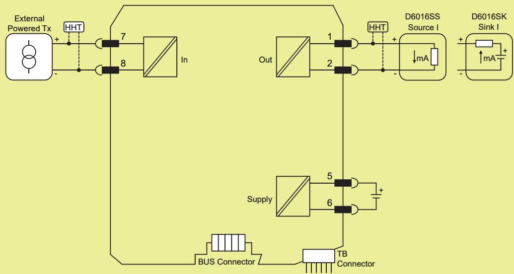
D6016S*
